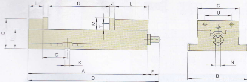
ATW/ATD DIMENSIONS
